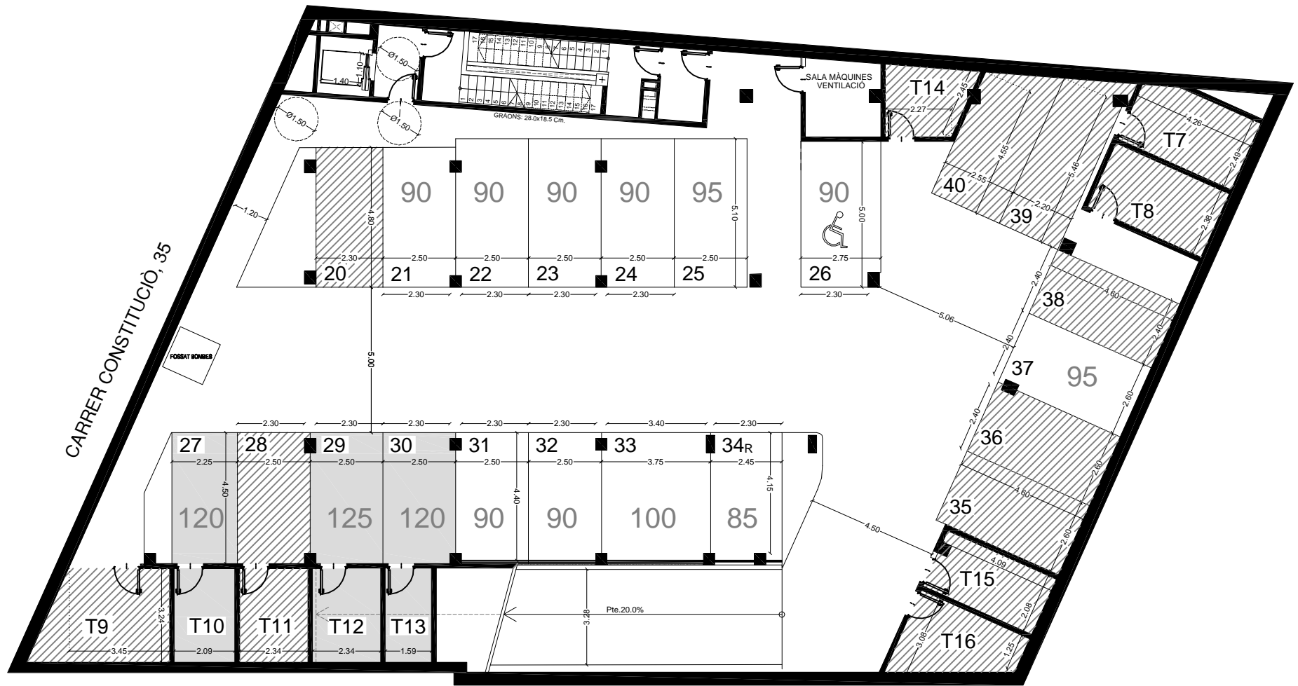
PLANTA SOTERRANI -2
