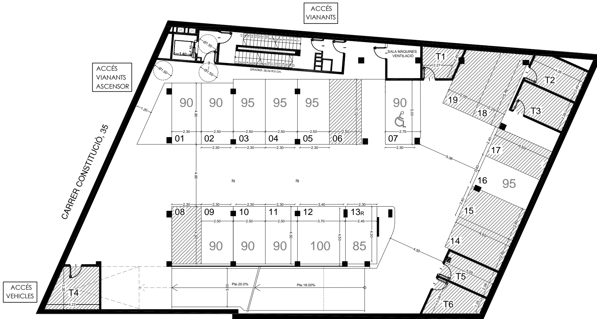
PLANTA SOTERRANI -1
